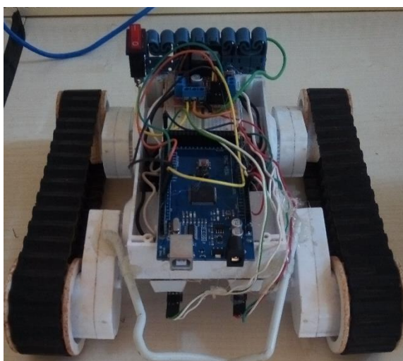
Figura 06 – Robô Seguidor de linha.
