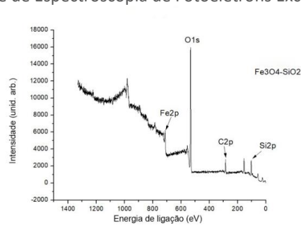
Figura 3 – Análise de Espectroscopia de Fotoelétrons Excitados por Raios X.
