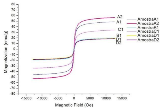
Figura 4 – Análise de Magnetometria de Amostra Vibrante.
