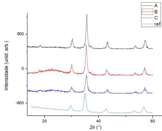
Figura 1 – Análise de Difração de Raios X.
